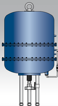
Doppel-Membranantrieb DMAA1.60
